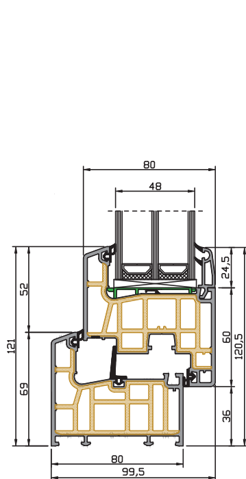
rama ze skrzydłem
