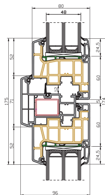
skrzydło ze słupkiem ruchomym
