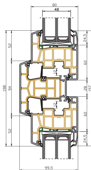
skrzydło ze słupkiem stałym
